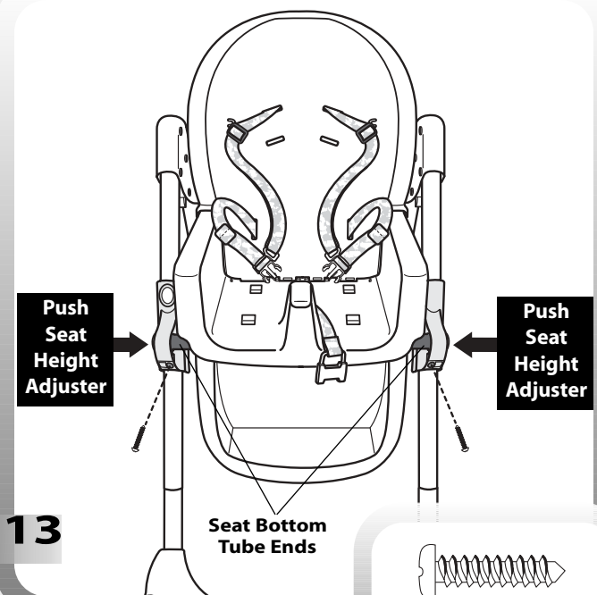
#8 x \frac{3}{4} " Screw - 2 SHOWN ACTUAL SIZE
